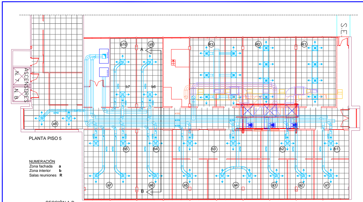
Plano distribución conductos
