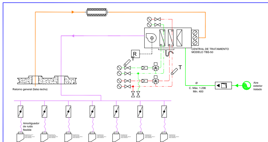
Plano distribución conductos
